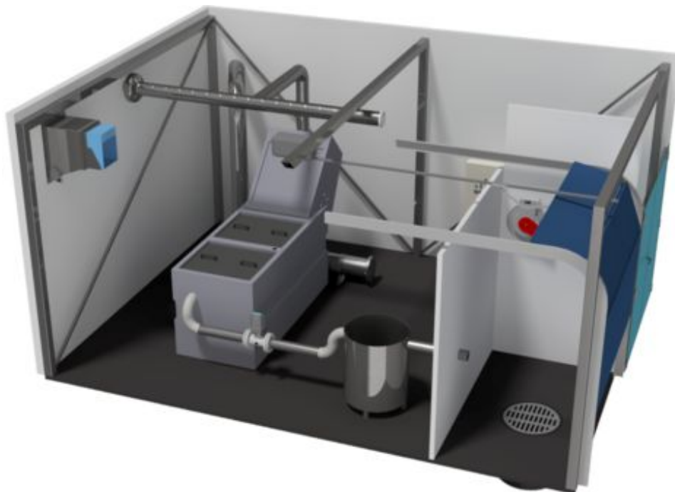
Система улавливания осадка из септика
