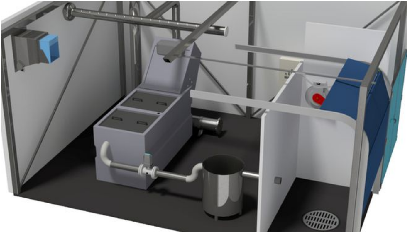
Система улавливания осадка из септика
